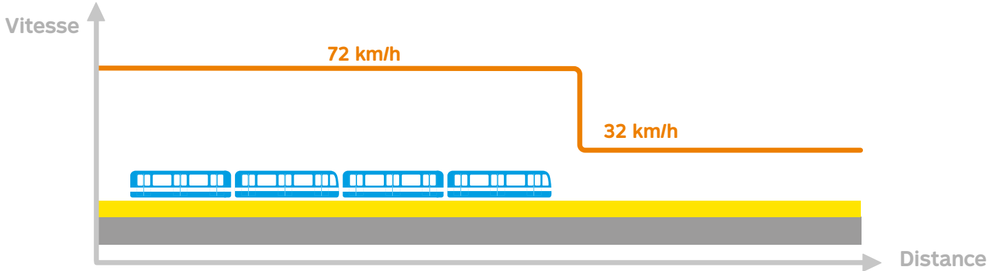
Courbe de freinage actuelle
