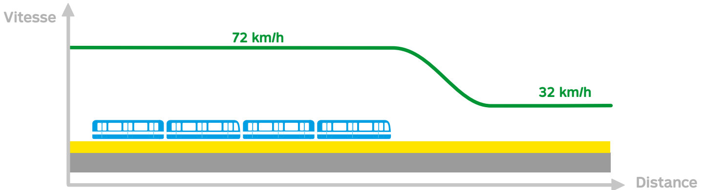
Courbe de freinage avec le nouveau système
