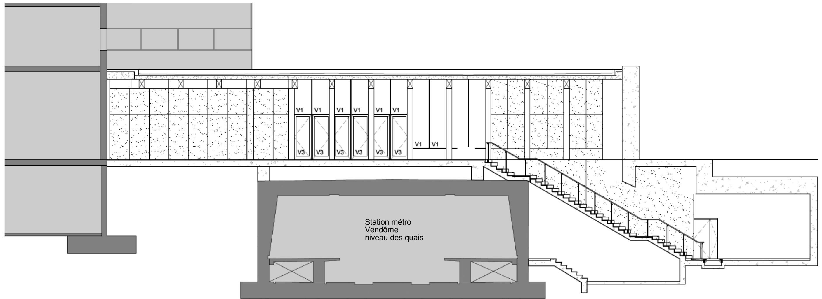
Coupe longitudinale au-dessus de la station de métro
